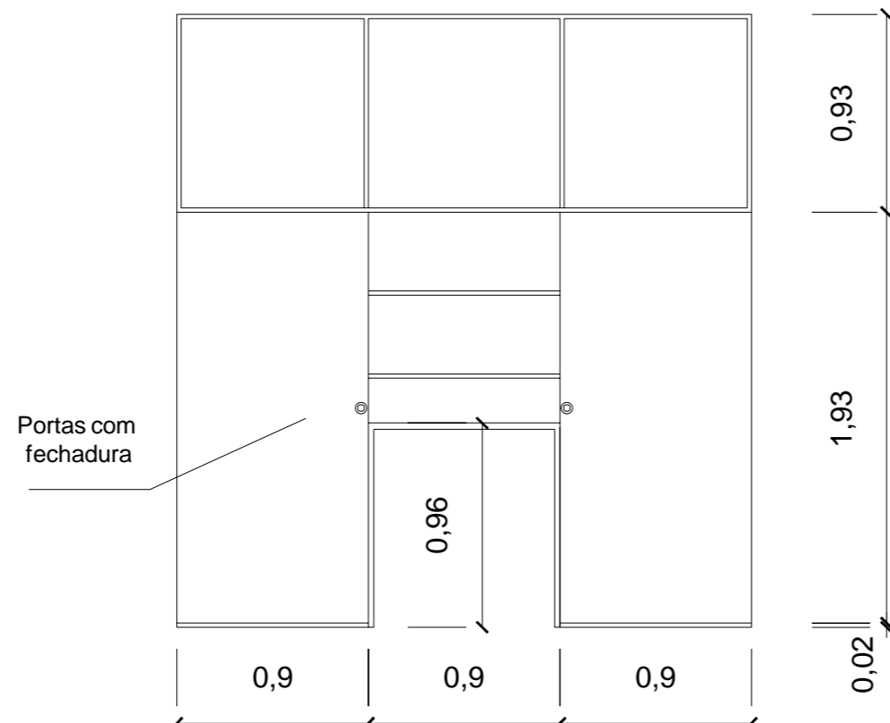
Vista Frontal- Portas Fechadas
