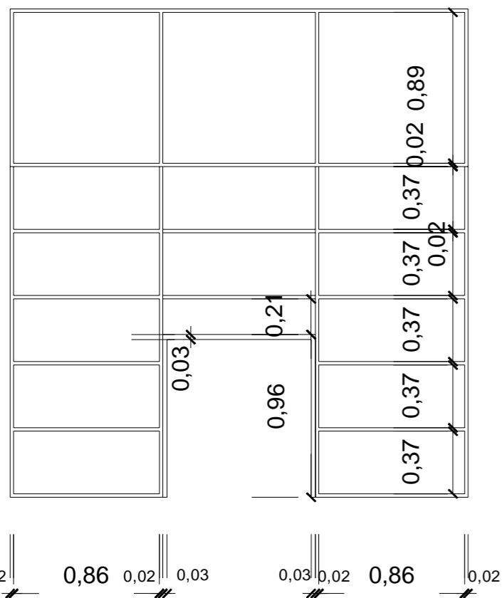
Vista Frontal- Portas Abertas, parte interna
