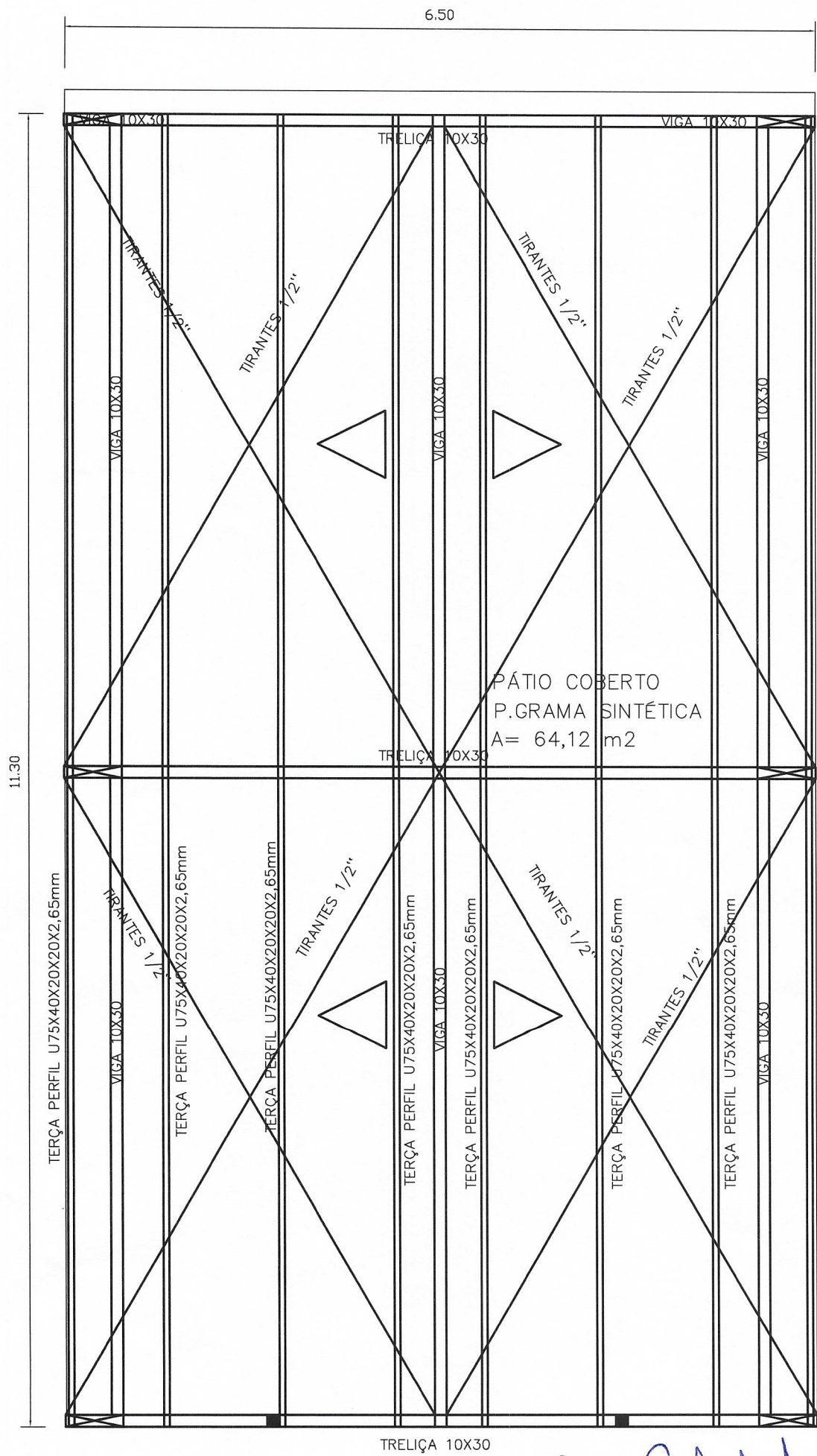
PLANTA COBERTURA
