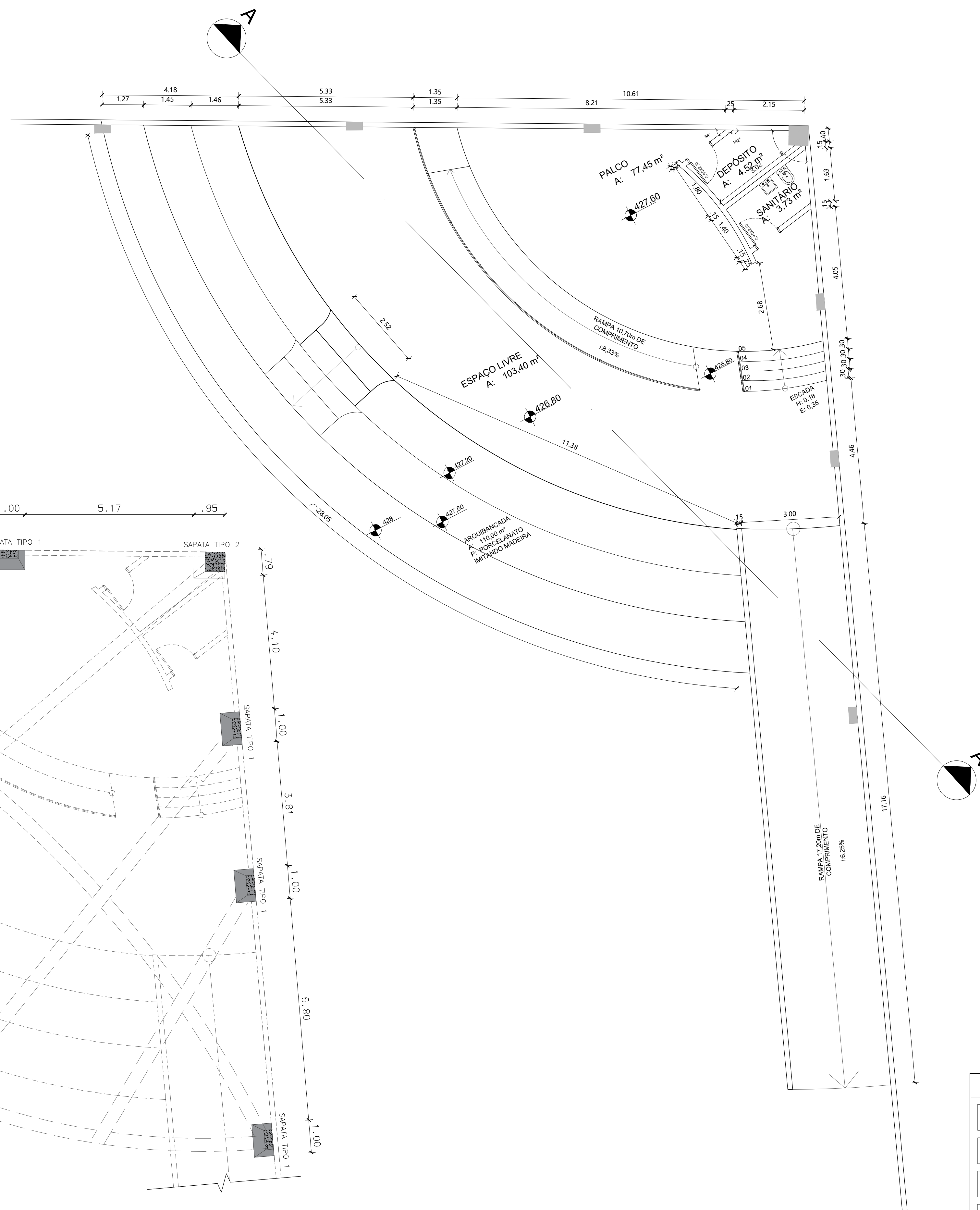
PLANTA BAIXA ESCALA 1/75
