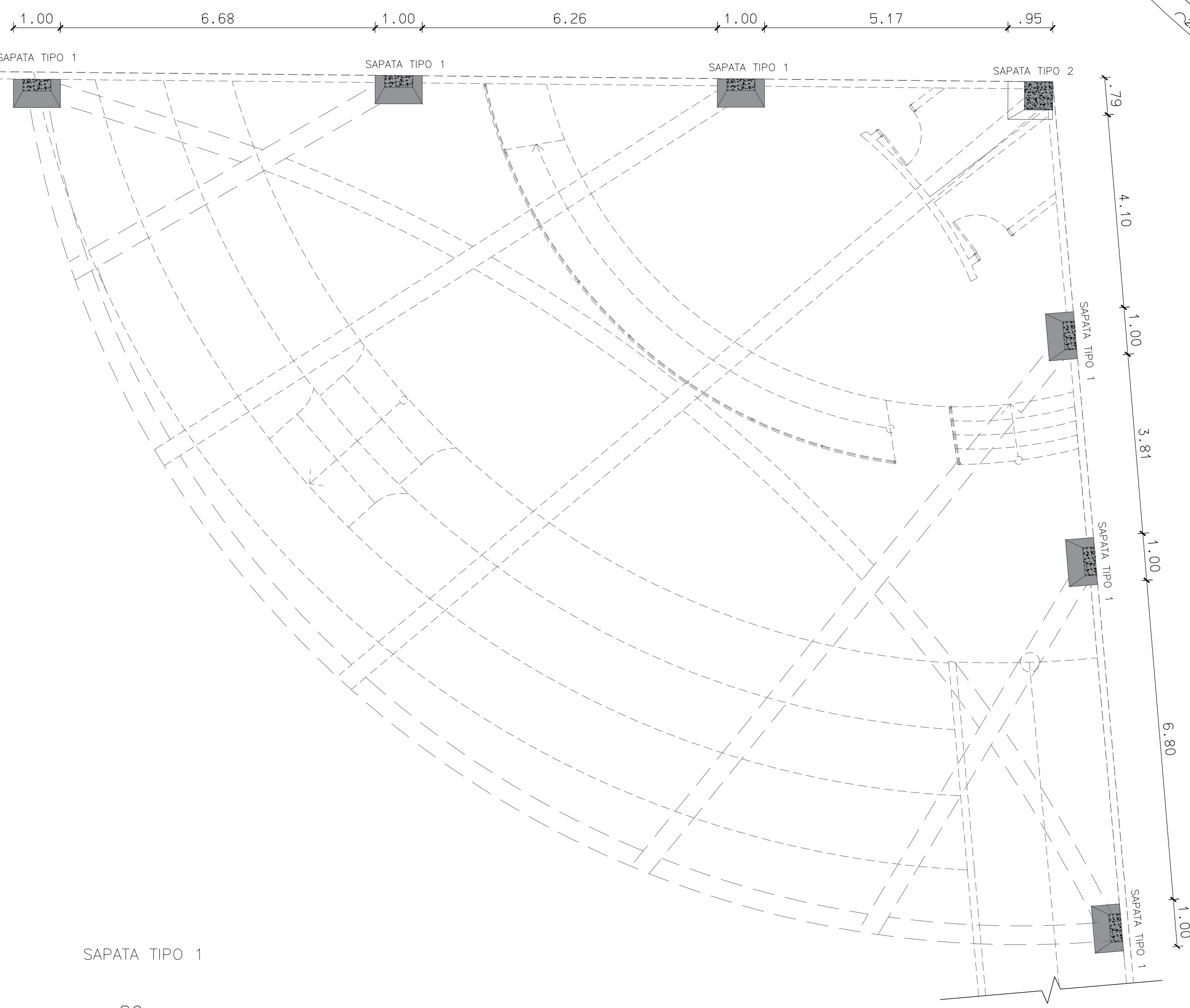
PLANTA SAPATAS ESCALA 1/75
